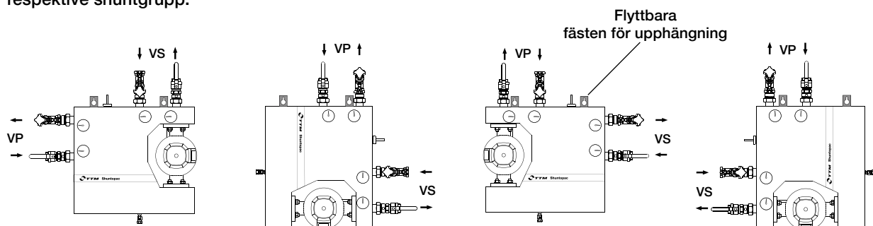
Monteringsexempel med TTM Shuntopac® 20-50 V.
