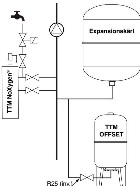
TTM Offset utjämningskärl
